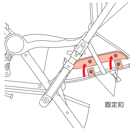
⑦ 解開靠背側邊的固定扣。(左右)
